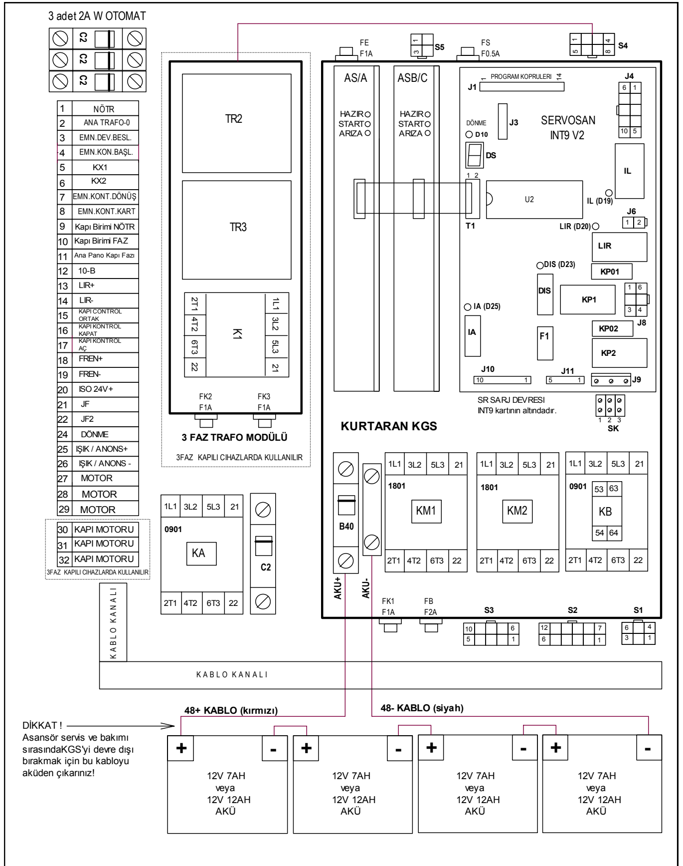
Şekil 1.PANOLU KGS16 YERLEŞİM ŞEMASI
